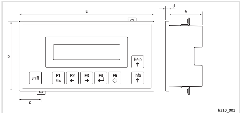
Abb. 2-2 Abmessungen
