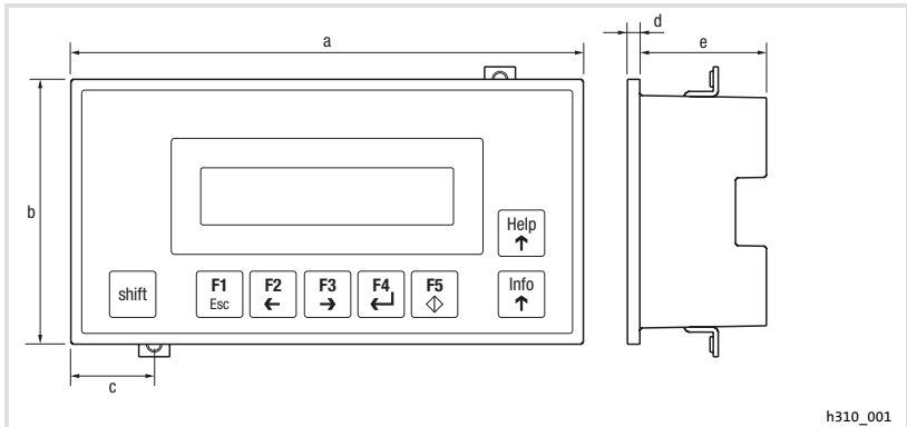
Fig. 2-2 Dimensions
