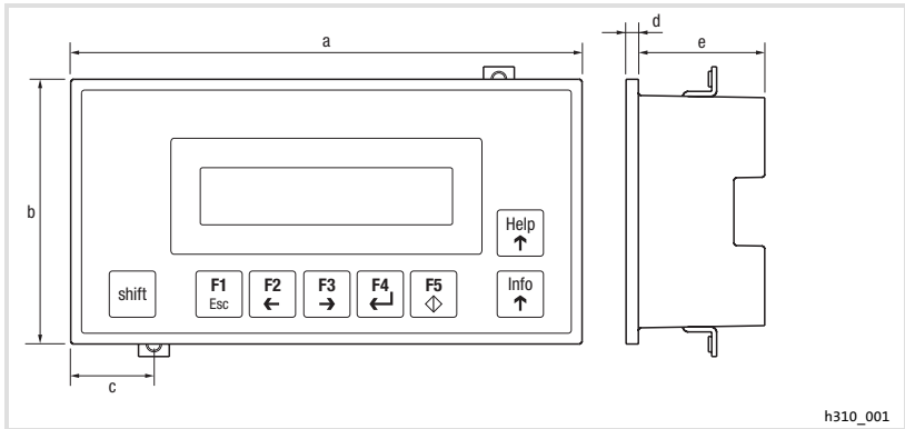
Fig.2-2 Encombremments
